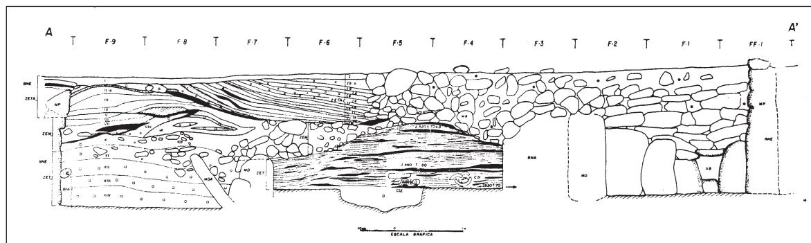
Figura 4. Perfil A-A' del sector nuclear del montículo excavado: MP, muro periférico; MDA, muro divisorio abatido; BNA, bloque no excavado; MD, muro divisorio; C, poste de cardón; BNE, bloque no excavado; AB, acceso a bodega embovedada; • muro abatido en sedimento eólico y cenizas (MA); D, depresión semicircular central; CI1, cuerpo neonato individual 1; CI2, cuerpo neonato individual 2 con ofrendas de iconos de oro; //// piso original de los recintos del módulo habitacional. ZET, zona estratigráfica temprana (datada entre 2630 a 2420 años a.P.); ZEM, zona estratigráfica media; ZETA, zona estratigráfica tardía.
