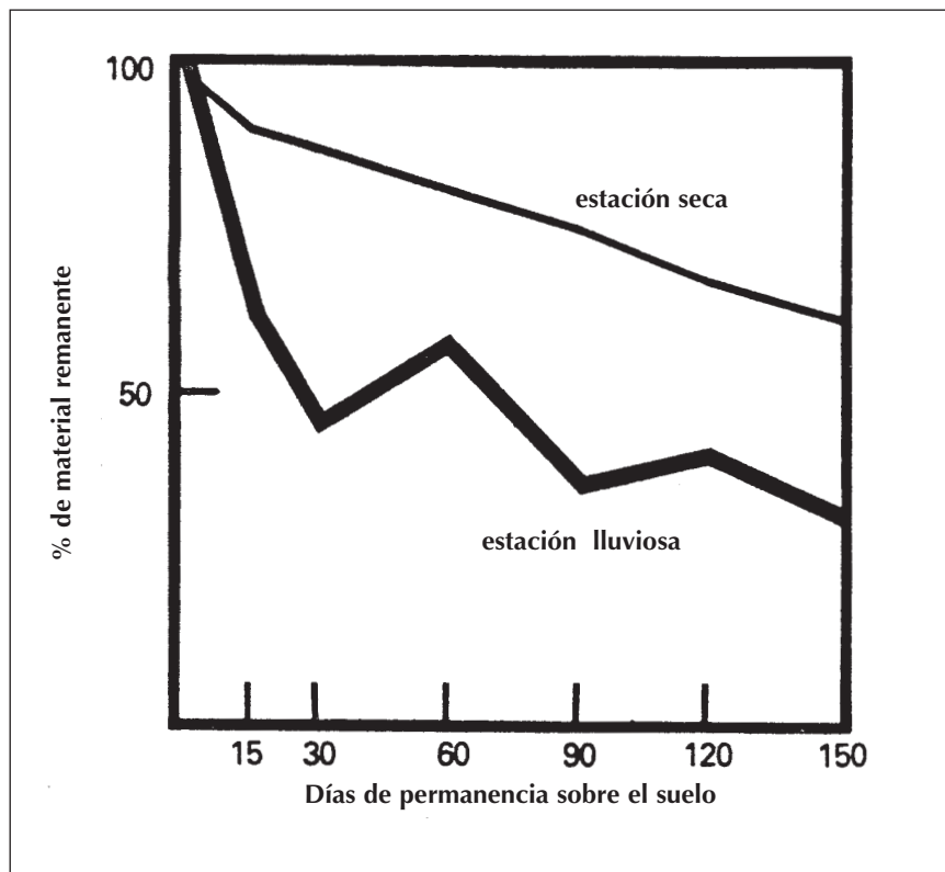
Figura. 3. Velocidad de descomposición de hojas muertas sobre el suelo durante la estación seca y la estación lluviosa. En la estación lluviosa después de 30 días el 50% de las hojas se encuentran bastante destruidas (según Schubart y otros 1984).
