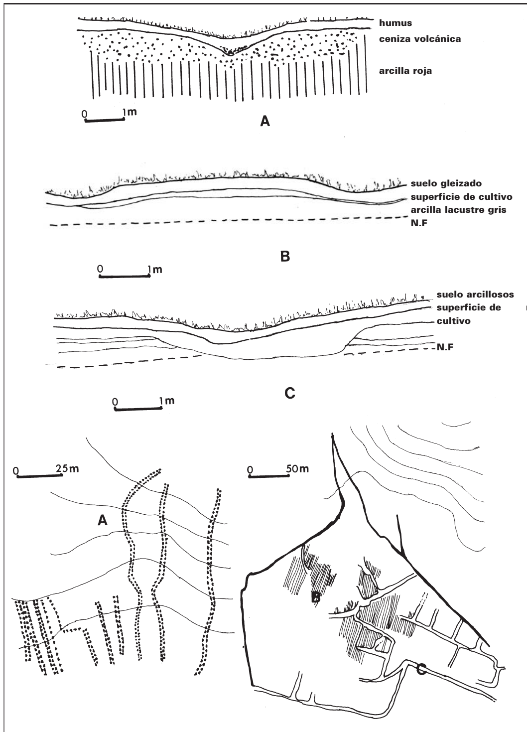
Figura 3. Adecuaciones agrícolas. En la parte superior se representan los cortes transversales y en la inferior las plantas de estas estructuras. A) canales en ladera. B) camellones y C) zanjás. N.F.= nivel freático (tomado de Herrera et al. 1990: figura 9)
